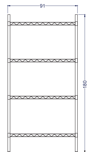
Vista Elevación
